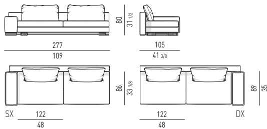
ELEMENTO TERMINALE CON BRACCIOLO CM 277 ELEMENT WITH ONE ARMREST CM 277
