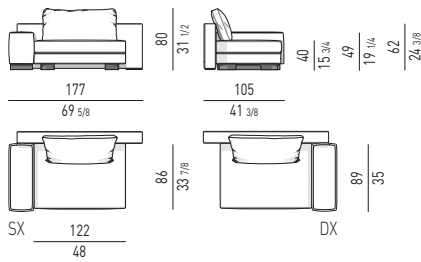
OFFSET ELEMENTO TERMINALE CON BRACCIOLO CM 177 OFFSET ELEMENT WITH ONE ARMREST CM 177
