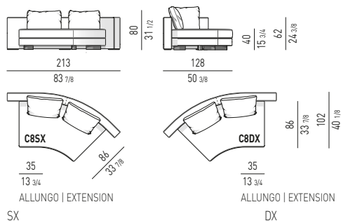
DOPIOFFSET ELEMENTO SEMICURVO CON ALLUNGO CM 213X128 DOPIOFFSET SEMI-ROUND ELEMENT WITH EXTENSION CM 213X128
